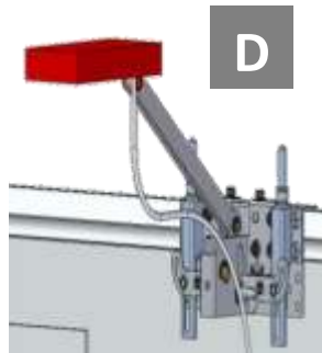
Dettaglio collegamento allo sblocco motore
