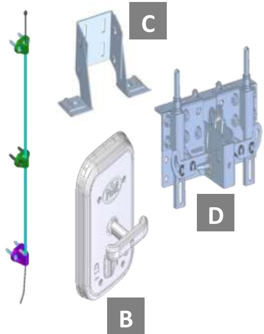
Gruppo serratura per apertura dall'esterno
